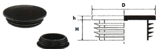
Tappo plastica nera per serie Ø33,7/Ø42,4
