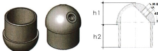
Base ang=45° ANTISCALATA per Perno M8
