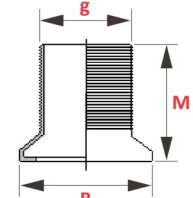
Semiraccordo con filetto maschio gas
