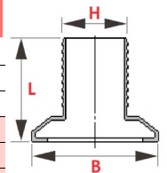
Portagomma ridotto
