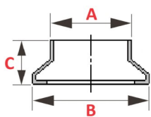
Semiraccordo a saldare
