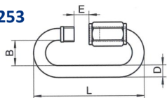
ANELLO CON APERTURA A VITE A.316
