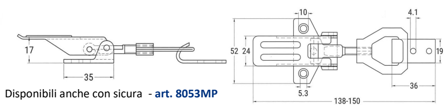
CHIUSURA A LEVA REGOLABILE TIPO M - A.304 art. 8053M
