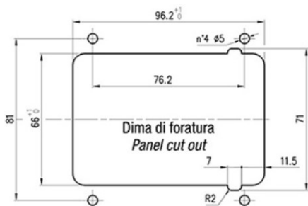
CHIUSURA A INCASSO CON SERRATURA - A.304 art. CH5S
