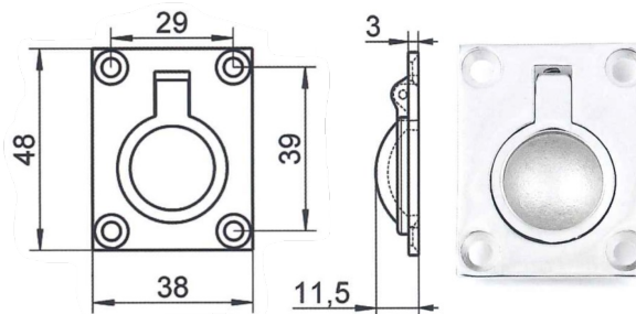
ALZAPAILO CON ANELLO MICROFUSO - A.316 art. 8243
