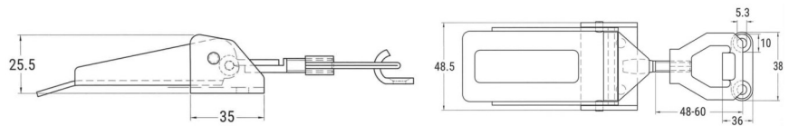
CHIUSURA A LEVA REGOLABILE TIPO L - A.304 art. 8053L
