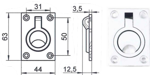
ALZAPAILO CON ANELLO ROBUSTO MICROFUSO - A.316 art. 8242
