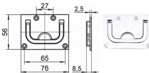
ALZAPAILO CON ANELLO MICROFUSO - A.316 art. 8243
