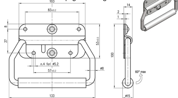
MANIGLIA PER CASSE CON MOLLA - A.304 art. FE770A
