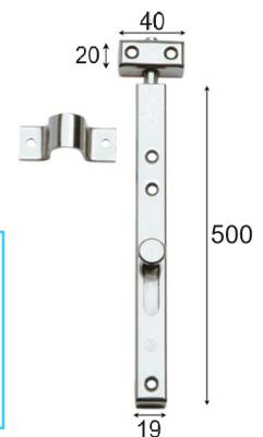
CATENACCIO VERTICALE CON FORI E FINALE TONDO A.304 art. 8117Q
