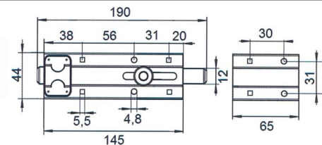
CATENACCIO TRASVERSALE ASTA PIATTA A.304 art. 8117M
