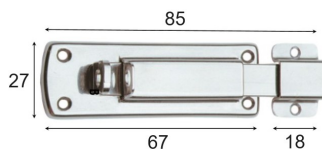
CATENACCIO TRASVERSALE ASTA PIATTA A.304 art. 8117L
