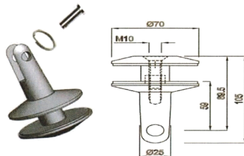
Fissaggio vetro inferiore
