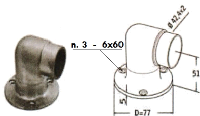
Piastra laterale corta
