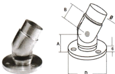
Piastra-attacco a muro con snodo
