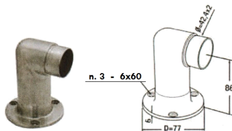
Piastra laterale lunga
