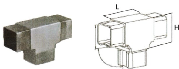
Pezzo a TEE
