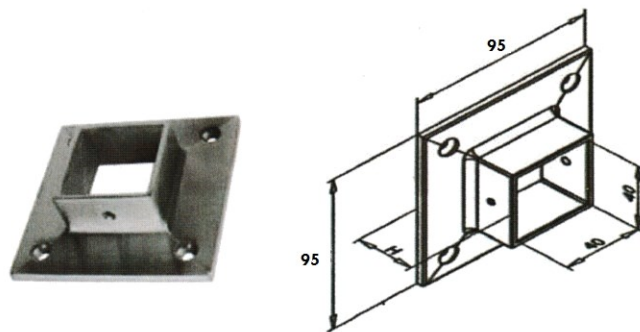
Flangia terminale a parete
