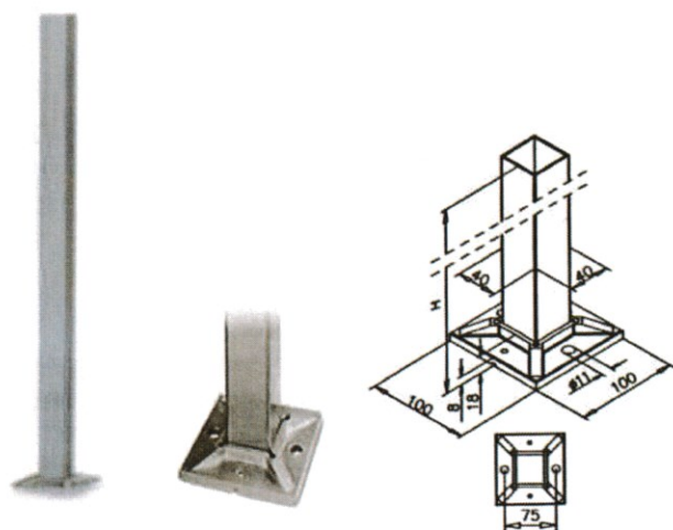
Montante quadro completo di Piastra 100x100mm
