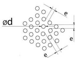
DETTAGLIO MAGLIA FILTRANTE
